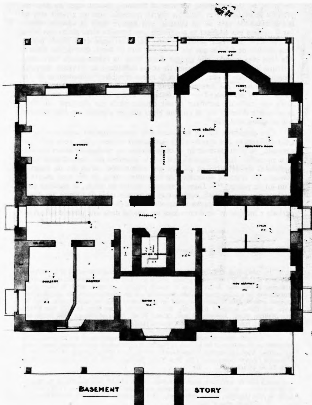
Illustration 2. — PLAN DU SOUS-SOL DE LA MAISON D'ANDREW THOMSON À QUÉBEC, 1860.
